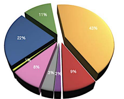
Figura 3.10.2. Ripartizione percentuale dell'emissione di \text{CH}_4 per le diverse specie allevate
