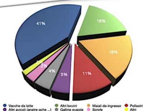
Figura 3.10.1. Ripartizione percentuale dell'emissione di \text{NH}_3 per le diverse specie allevate
